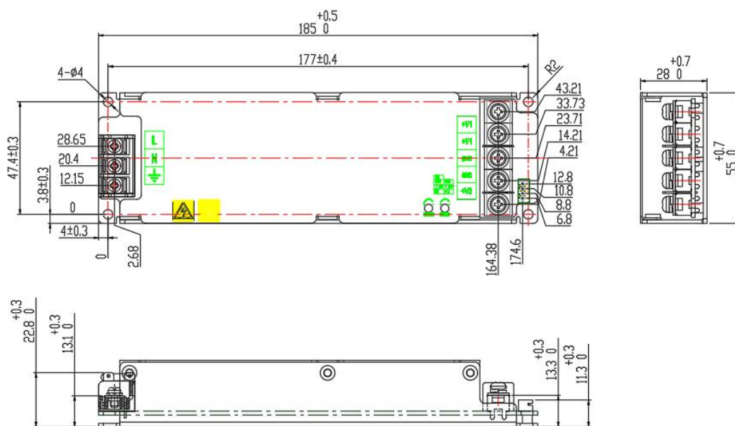
外形尺寸及安装孔——端子坐标图
